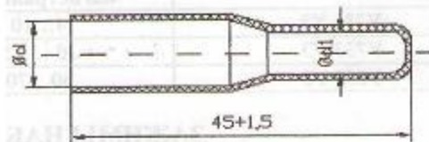
Рис. 1 Колпачки К440, К441, К444
